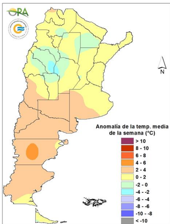
Anomalía de la temperatura media de la semana del 23/10/2024 al 29/10/2024
