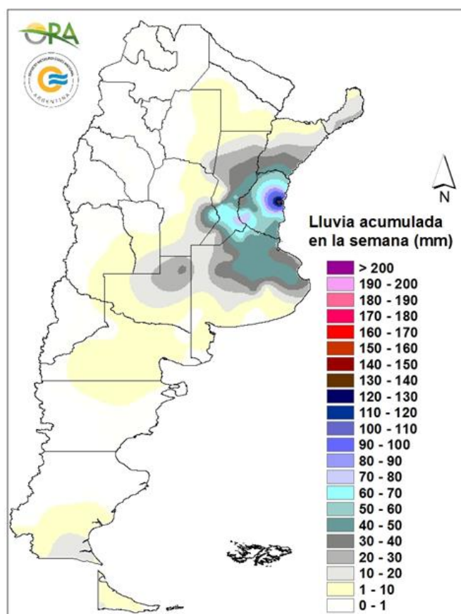
Precipitaciones acumuladas en la semana del 23/10/2024 al 29/10/2024
